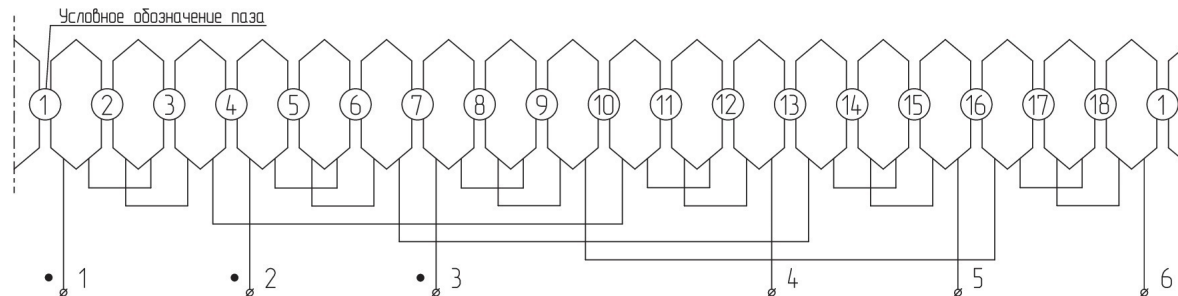
Схема обмотки
