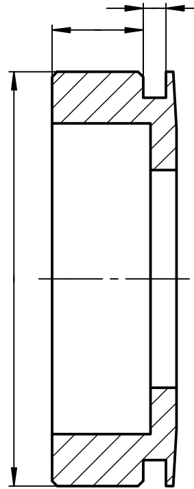
Ролик шестерни направляющий
