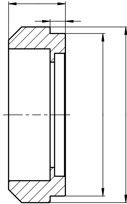
Ролик внутренний тип1
