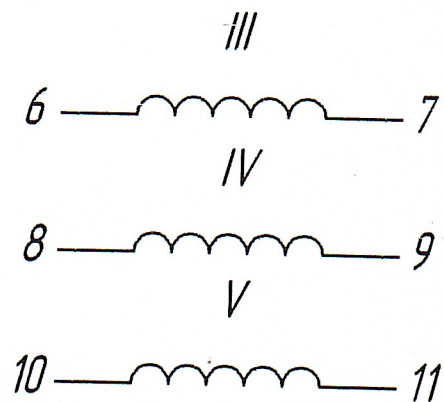
Схема обмотки
