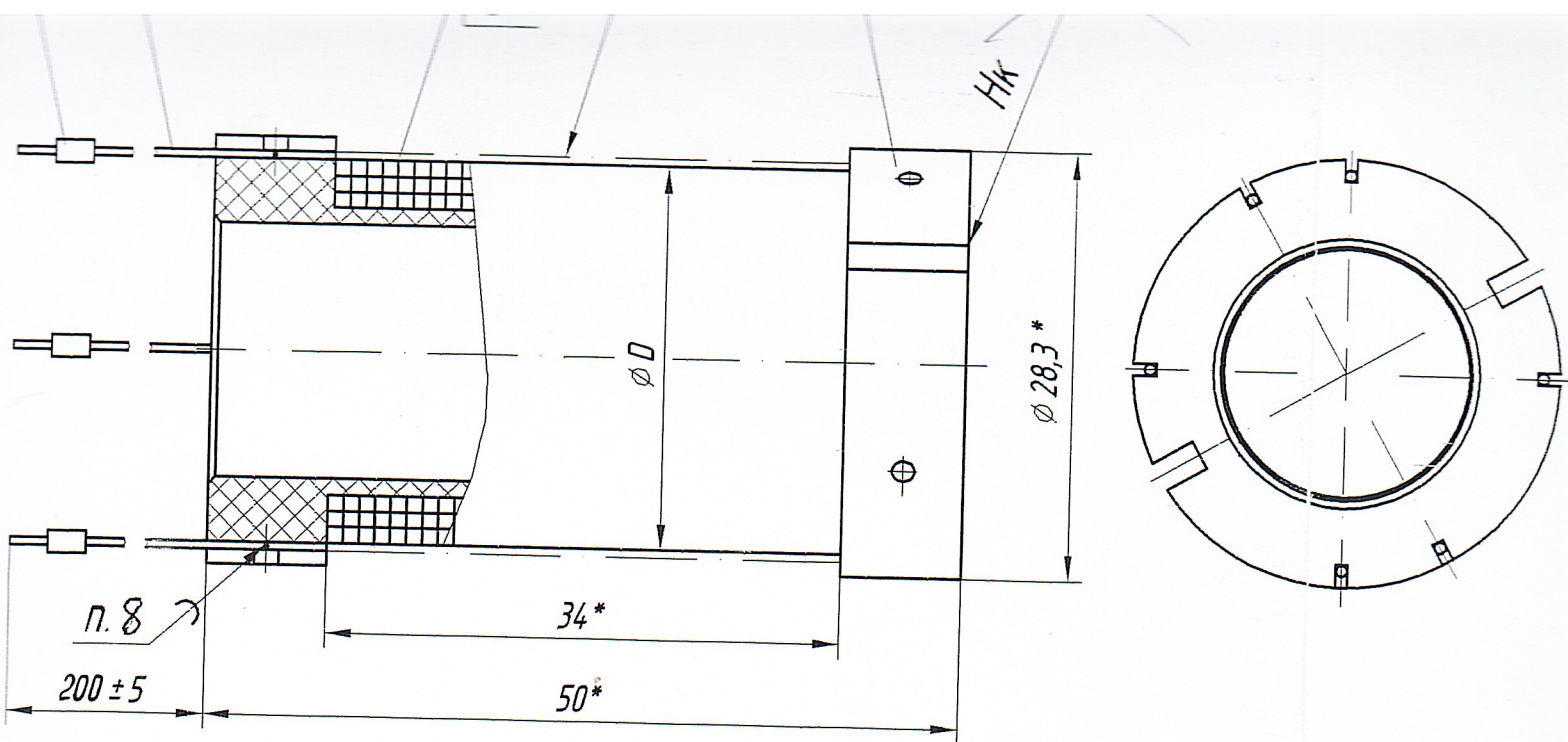
Схема обмотки
