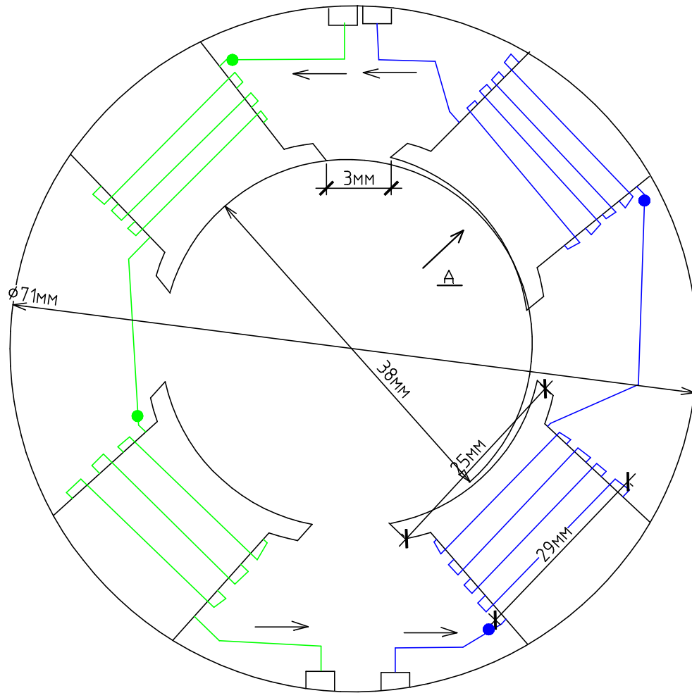
Вид А
