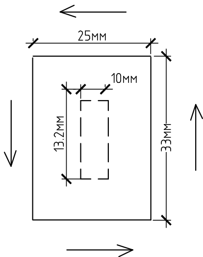
Вид А
