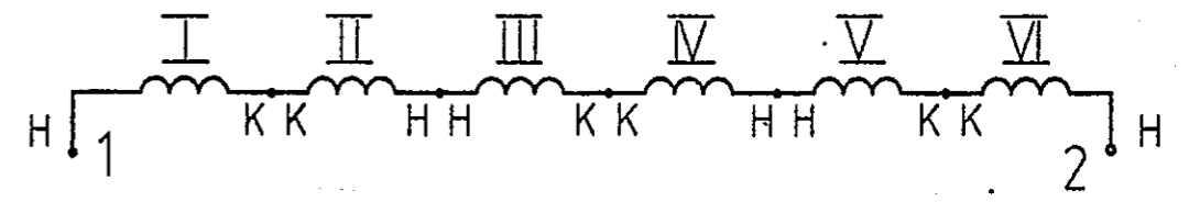
Схема электрическая
