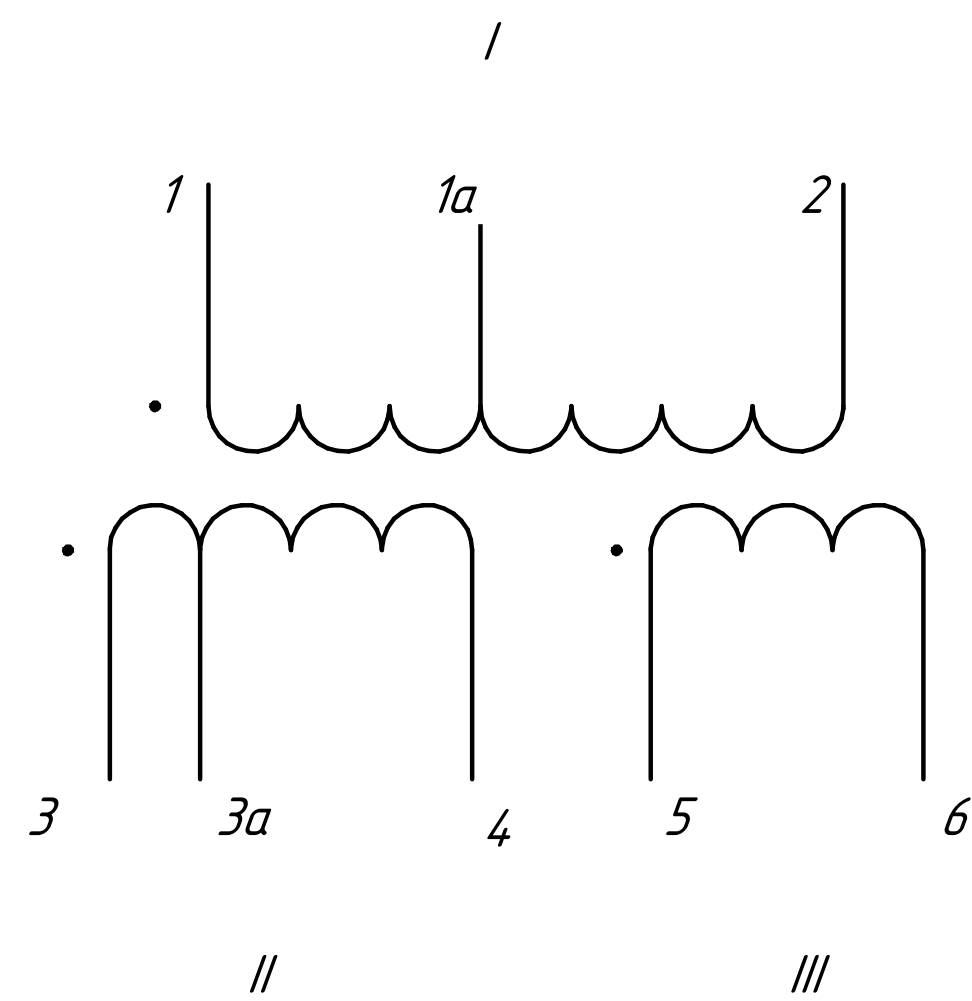
Схема обмоток
