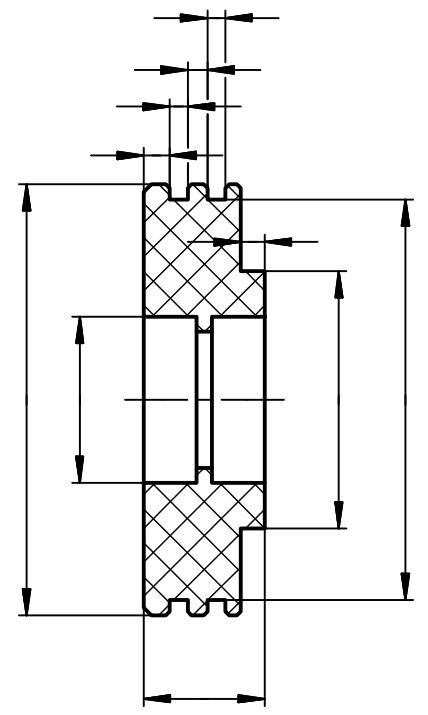
Ролик капролоновый
