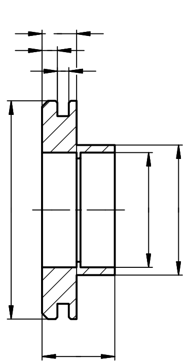
Ролик стальной
