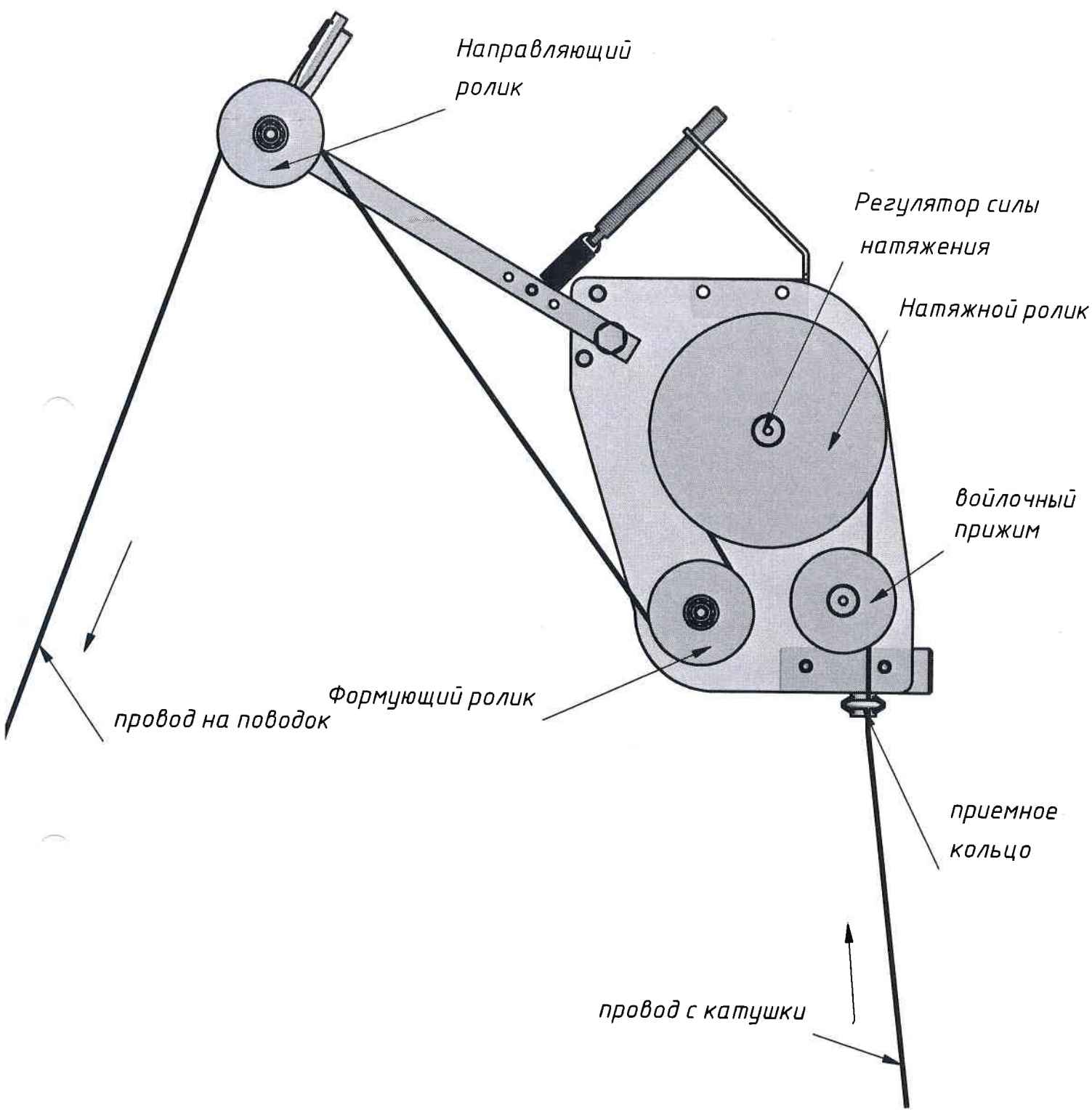
Пример заправки провода на ФНУ
