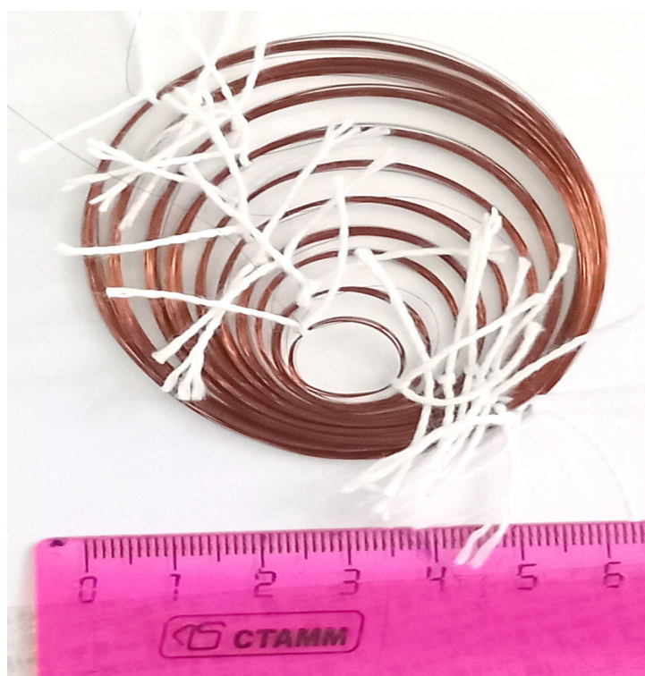
Намотанные секции.
