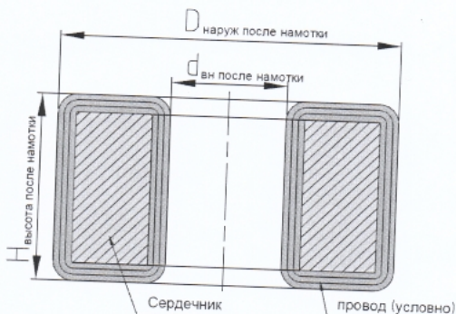
Рисунок 2. Сердечник после намотки
