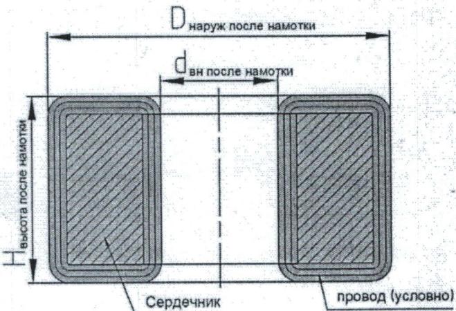
Рисунок 2. Сердечник после намотки
