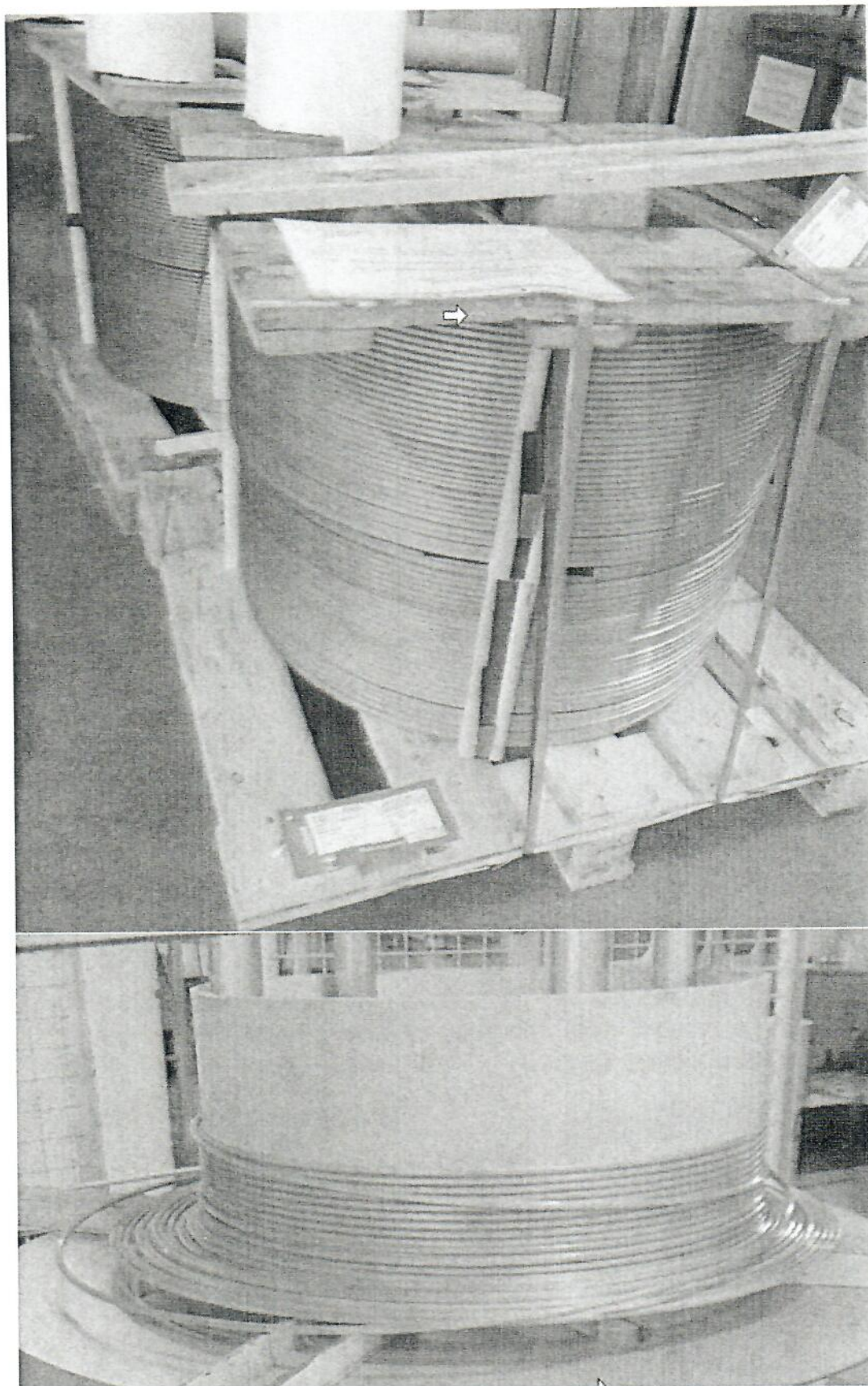
Пример упаковки бухт и намотки прутка
