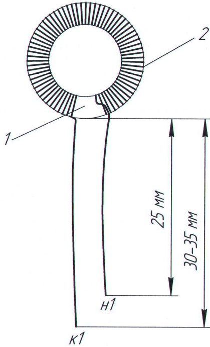
Трансформатор Т1 (токовый)
