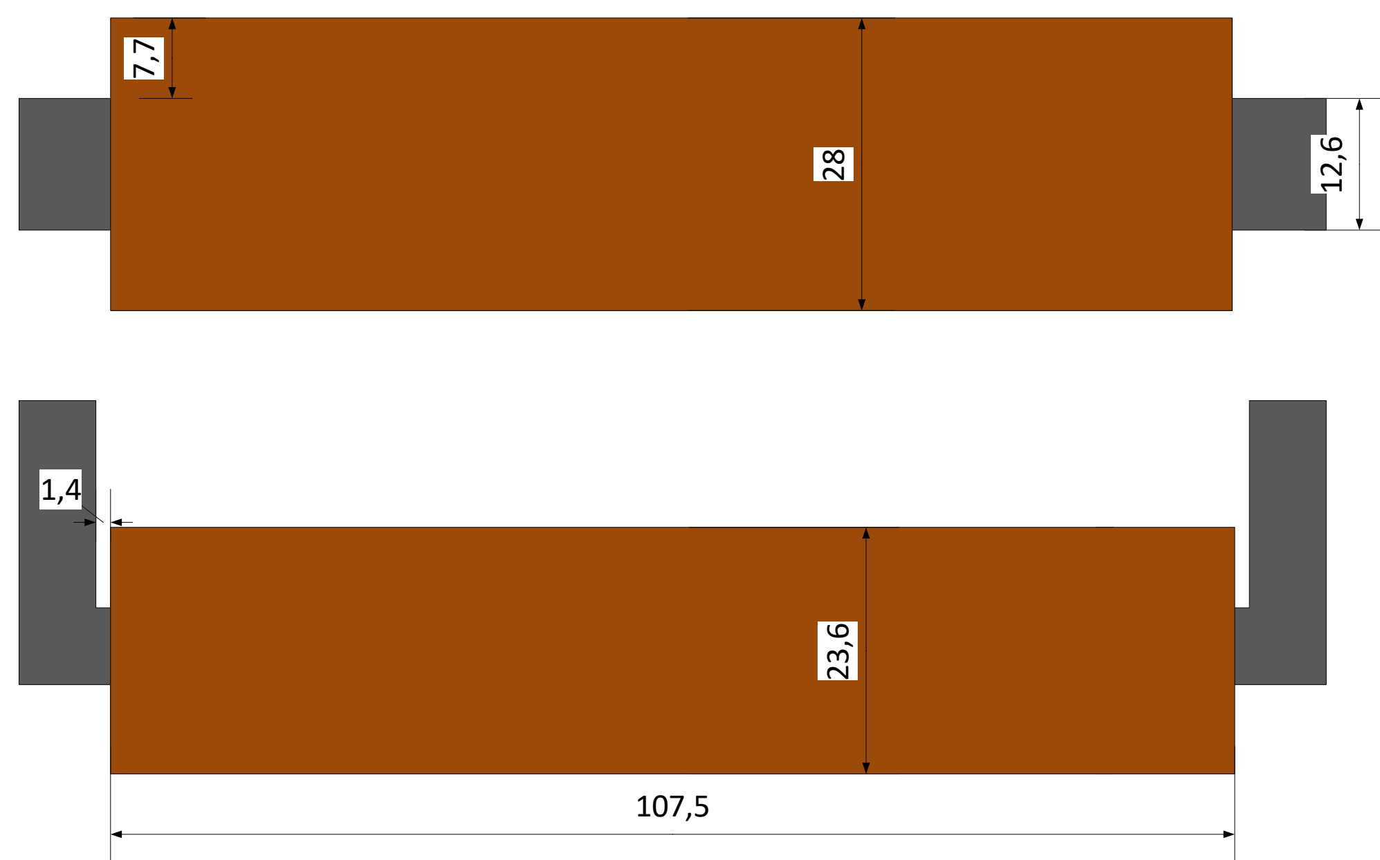
Катушка ТТ 2000 А
