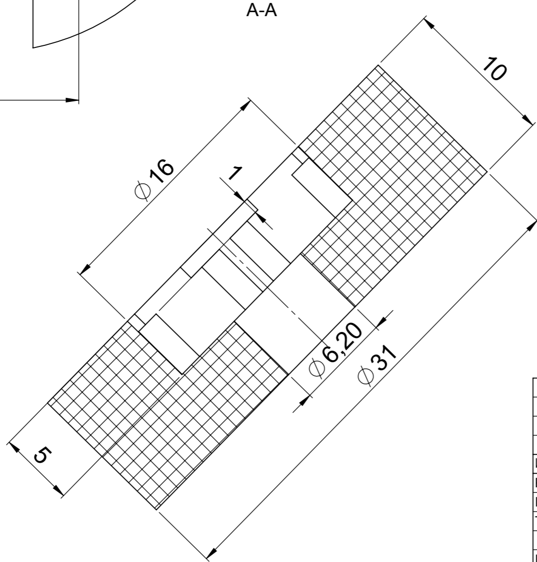
1. Размеры для справок.
