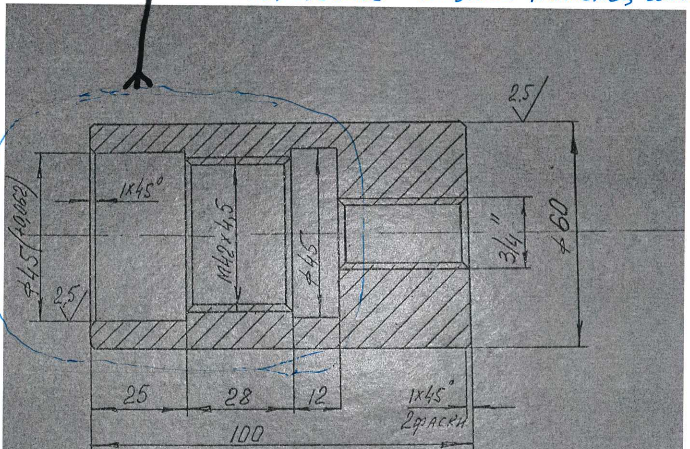
Переходная втулка на конец шпинделя
