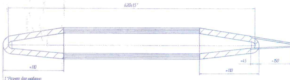
Эскиз № 1 (секция).
