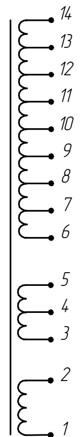
Электрическая схема трансформатора
