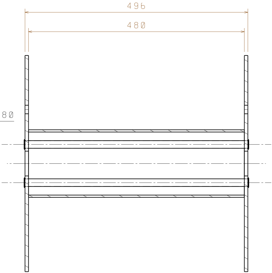
Вид спереди Масштаб: 1:4
