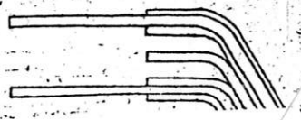
Вид Г развёрнуто M25:1
