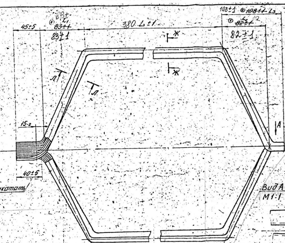
Вид Г развёрнуто M25:1
