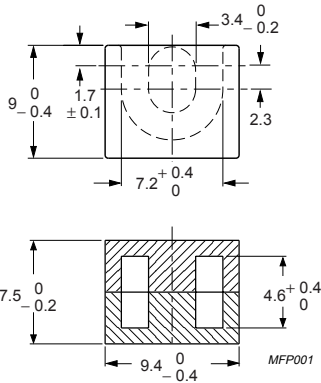
Fig.1 EPX7 core set.
