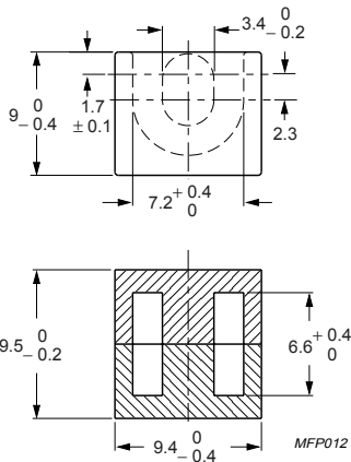
Fig.1 EPX9 core set.
