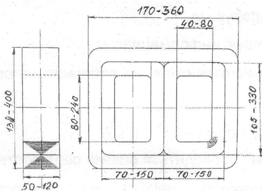
Рис.1. МП для 3-х фазного трансформатора. - толщина эл.- техн. стали – 0,3 мм; - ширина полосы – 50-120 мм; - рулон d_{вн} \times d_{нар} = 500 \times 1000 мм; - вес рулона -135-600 кг.
