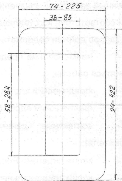
Рис.2. МП для однофазного трансформатора. - толщина эл.- техн. стали – 0,3 мм; - ширина полосы – 30-135 мм;
