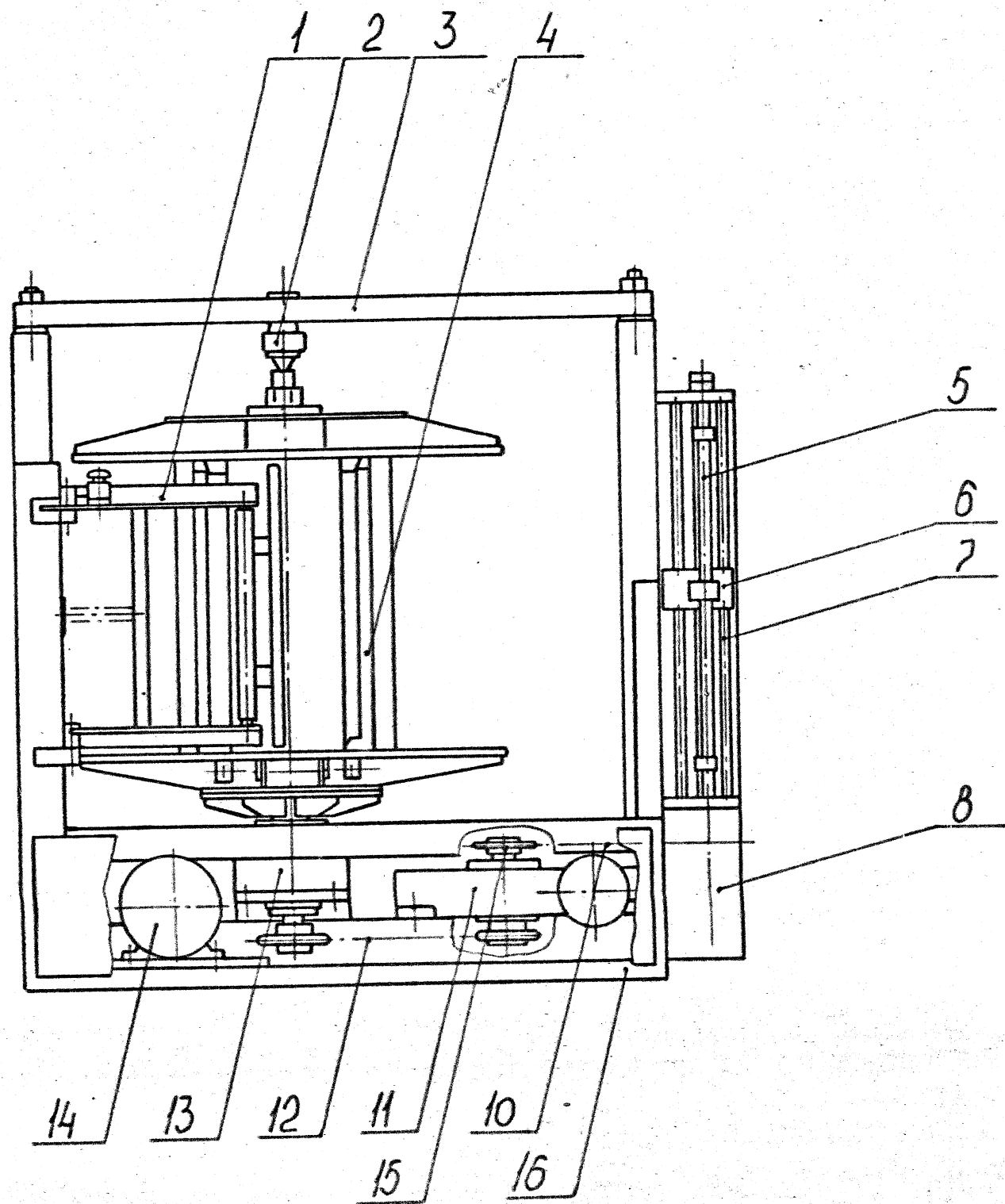
Рис. 1 Общий вид станка намотки проволоки.
