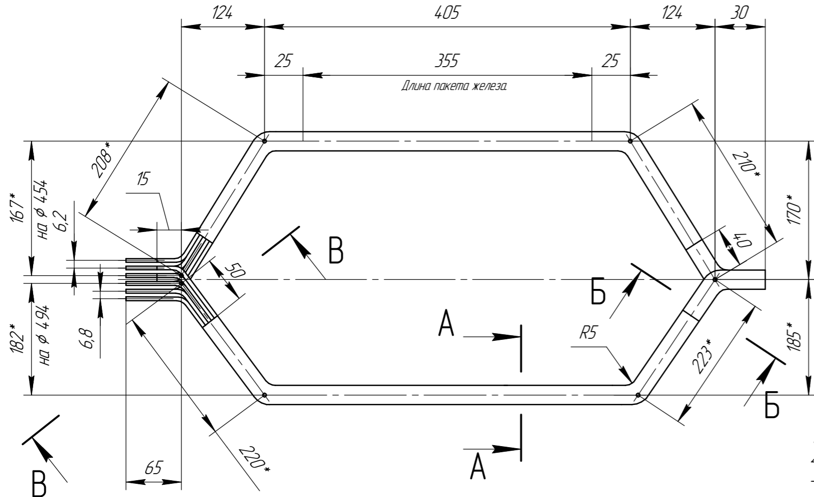
Размеры паза в свету.
